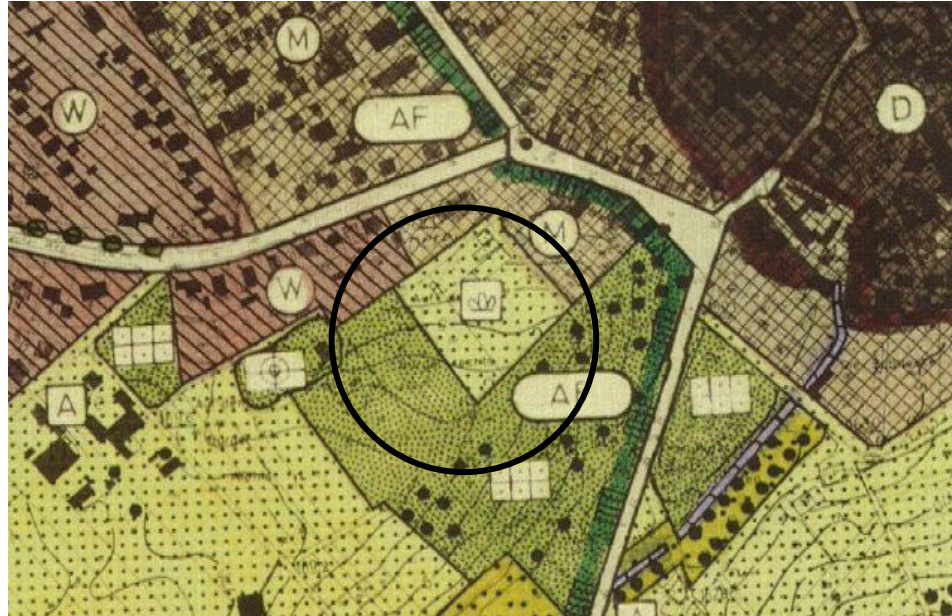
Abbildung 6: Ausschnitt aus dem Flächennutzungsplan mit Landschaftsplan (März 1990) der Gemeinde Schaafheim
